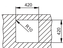
Hueco de encastre
