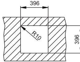
Hueco para montaje bajo encimera
